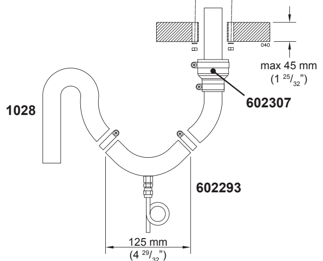
Suljettava kansiläpivienti 2466 asennus. Asennusaukko on \varnothing 50 mm ja ruuvien reiät 4 x \varnothing 6 mm.
