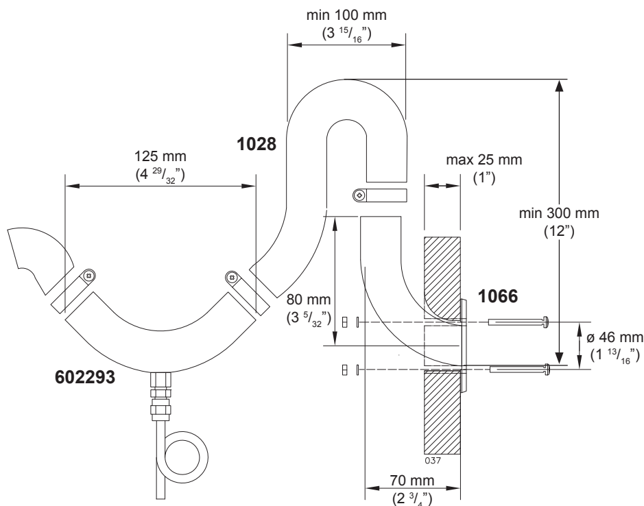
Installation av avgasgenomföring 1066 i skrovet. Monteringshållet ska vara \varnothing 35 mm och skruvhålen 4 x 5 mm.
