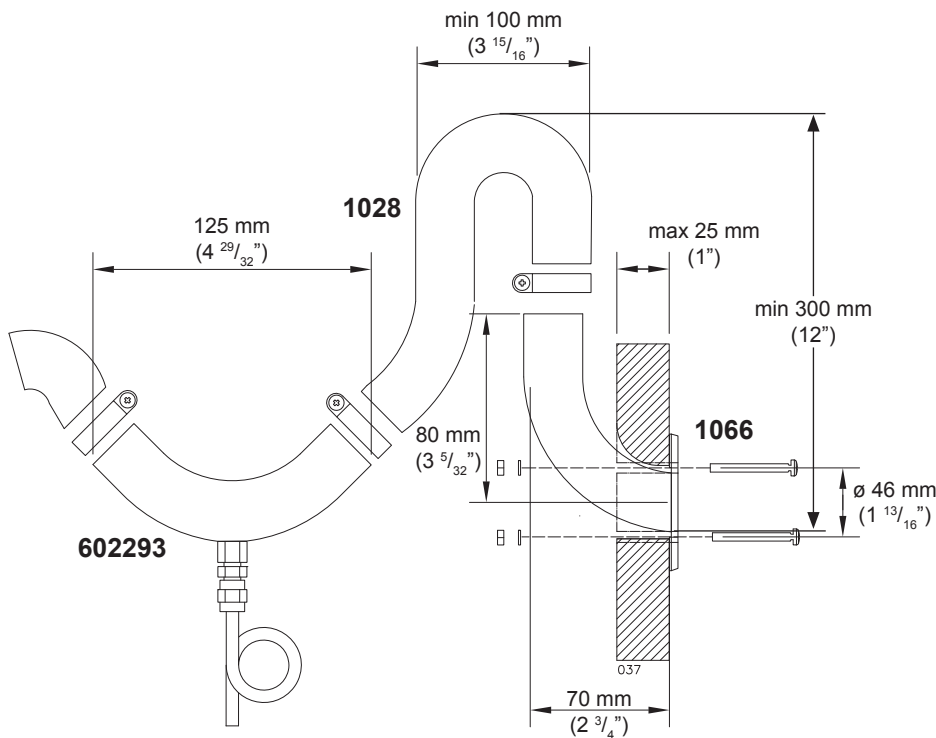
Installatie van spiegel/romp uitlaat 1066 in de romp. De installatie opening is \varnothing 35 mm en de schroefgaten zijn 4 \times \varnothing 5 mm.
