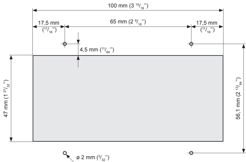
Mesures de l'échancrure de l'installation du panneau de contrôle Si nécessaire, faire des avant trous pour les vis de Ø 2 mm (3/32").
