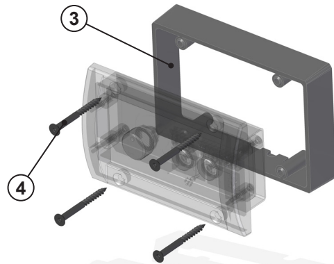
Un collier est utilisé pour installer le dispositif de commande sur une surface (3). Le kit contient 4 vis de fixation 3,5 x 40 mm (noir) TX10 (4).
