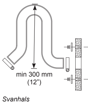
Svanhals
