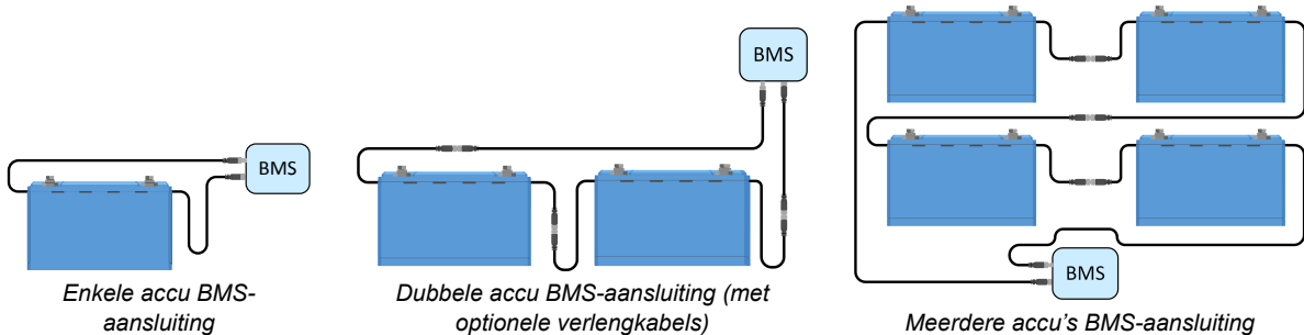
Meerdere accu's BMS-aansluiting
