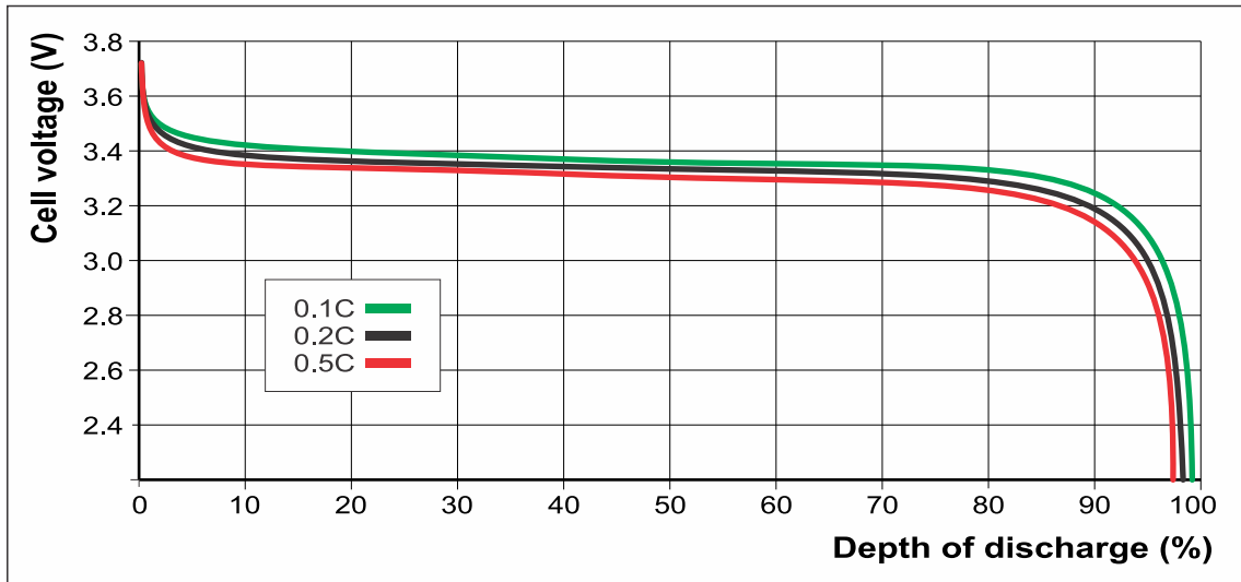
Ontlaadgrafiek die de celspanning laat zien voor verschillende ontladingsdieptes voor verschillende ontladingsnelheden
